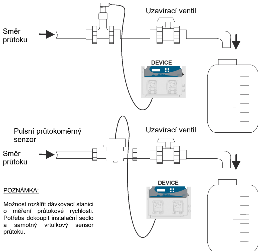
Mechanický (vrtulkový) průtokoměrný senzor
