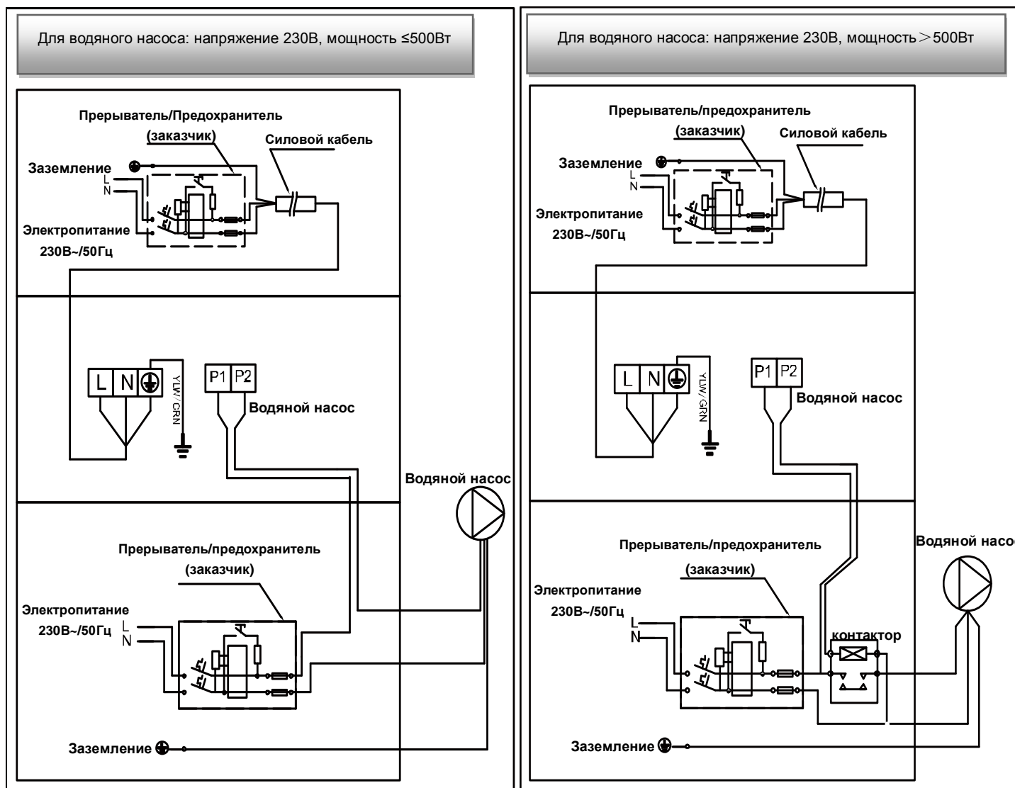
Приложение 1: Монтажная схема соединения приоритетности обогрева (опция)
