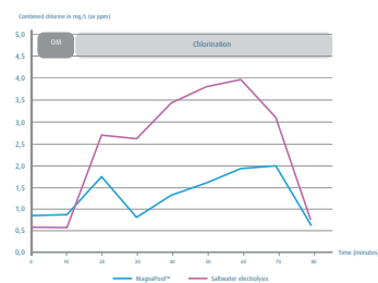
Křivka poklesu vázaného chlóru oproti slané vodě
