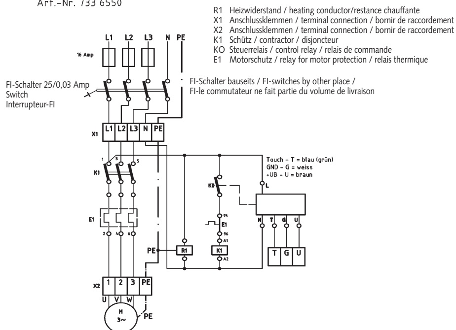
Schaltbild Sensorschaltung 400V / 3 N ~ mit Heizwiderstand 2,6kW DS Circuit diagram wiring Schéma de raccordement Art.-Nr. 733 6550
