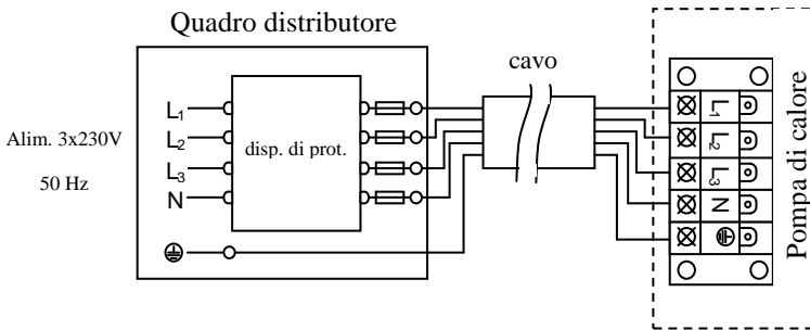
A. Schema collegamento elettrico da trifase 400 V 50Hz
